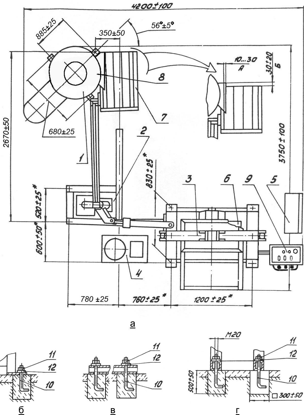
Рис. 1.1 Общая компоновка линии
